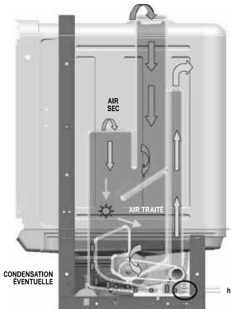
NOUVELLE POCHÉ DE SÉCHOIR
