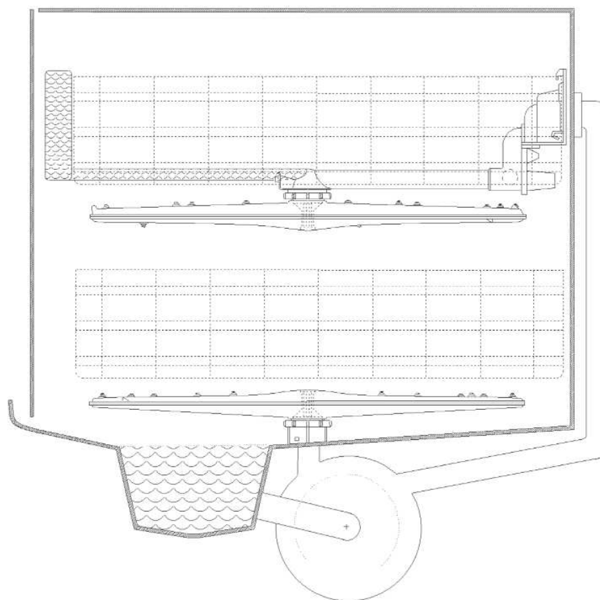
d) bras d'aspersion supérieur
